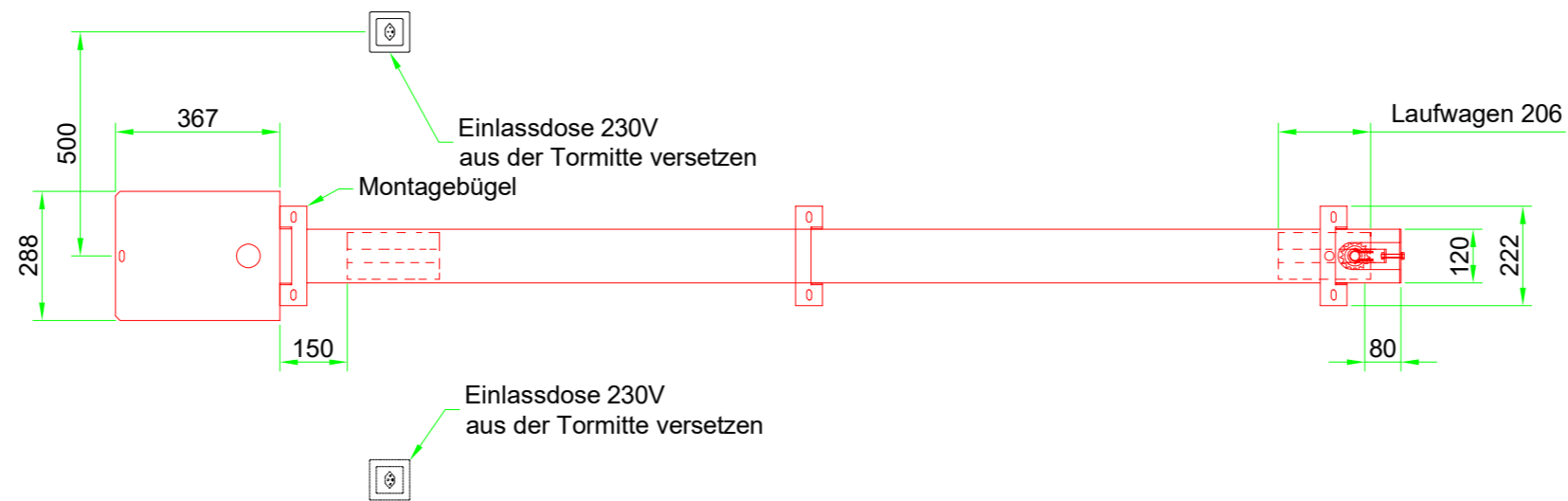
Ansicht Y
