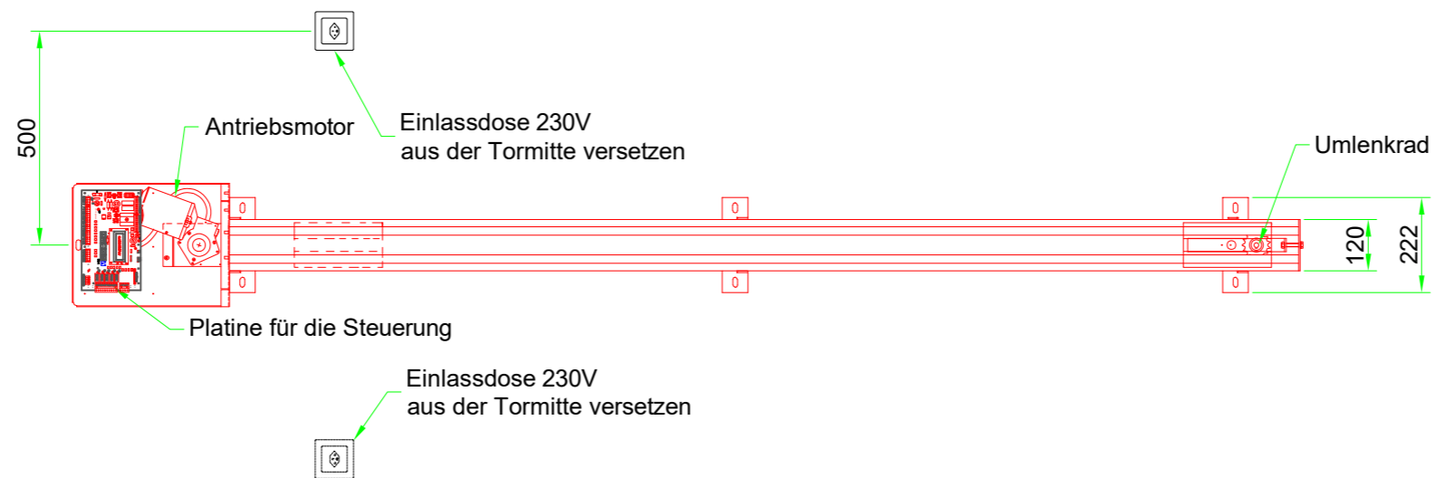
Ansicht X
