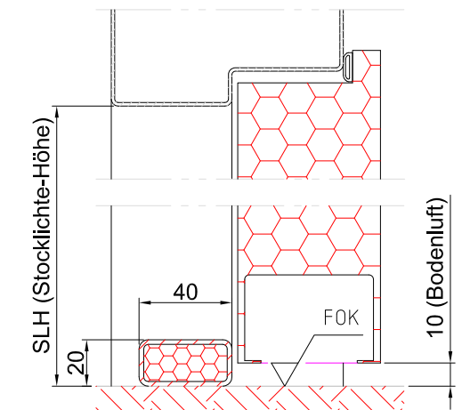
Aufbauschwelle Formrohr (20 mm) - Auswahl 2 Min. Bodeneinstand: ohne
