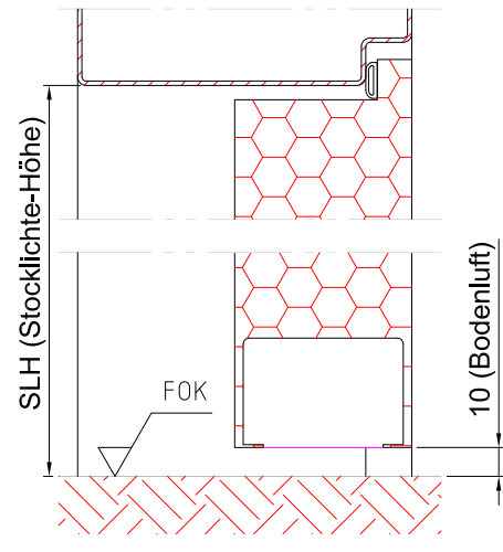
ohne Aufbauschwelle - Auswahl 0 Min. Bodeneinstand: ohne
