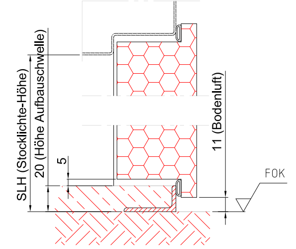
Aufbauschw.Winkel (20)+TB vierseitig-Ausw.11 Min. Bodeneinstand: ohne
