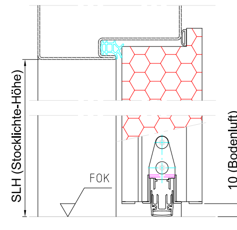
Absenkbare Bodendichtung Planet PU Beispiel Zarge mit Dichtnut, mit Bodentrennschiene
