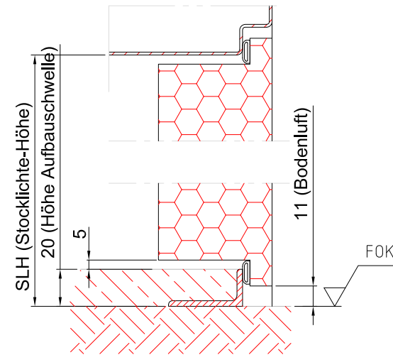
Aufbauschw.Winkel (20)+TB vierseitig-Ausw.11 Min. Bodeneinstand: ohne
